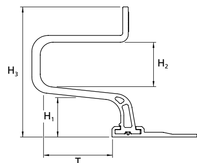
Bemaßungsschema SingleHook
