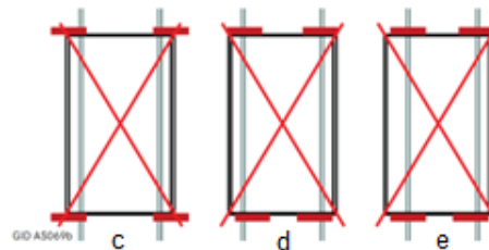
Abb. 7 Unzulässige Anordnung der Klemmen bei gerahmten Modulen (2)
