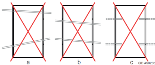
Abb. 4 Unzulässige Führung der Montageprofile
