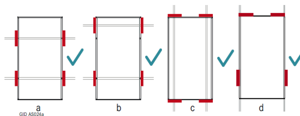
Abb. 5 Zulässige Anordnung der Klemmen bei gerahmten Modulen
