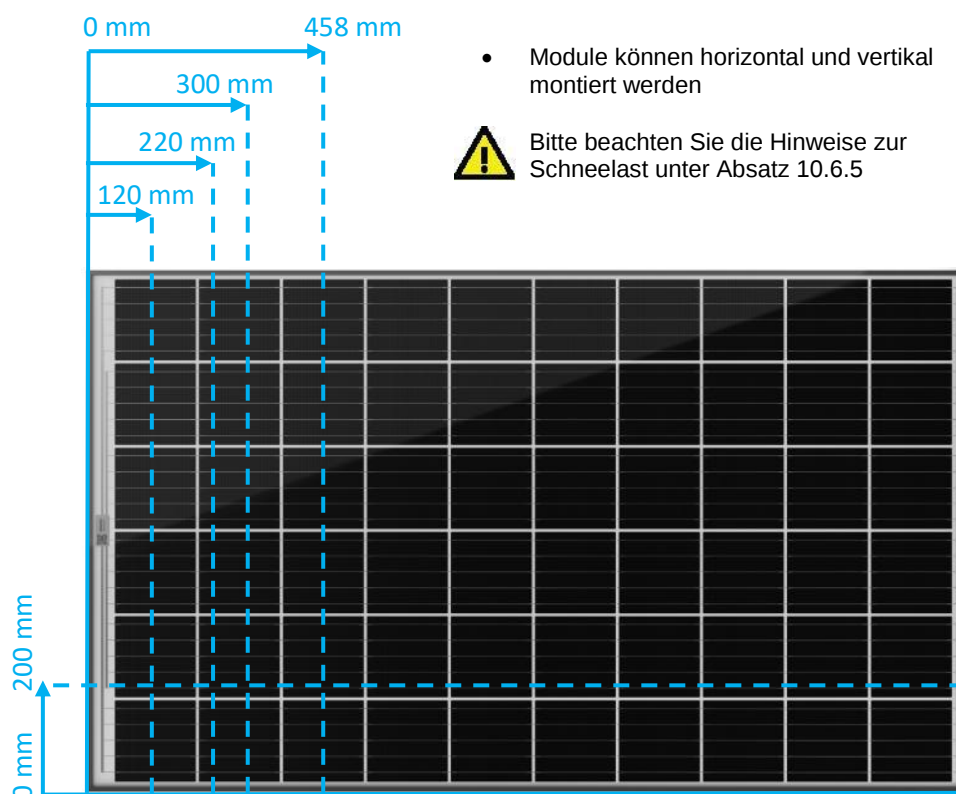
Abb. 9 Montage X63/ X83 Modul mit Klemmen
