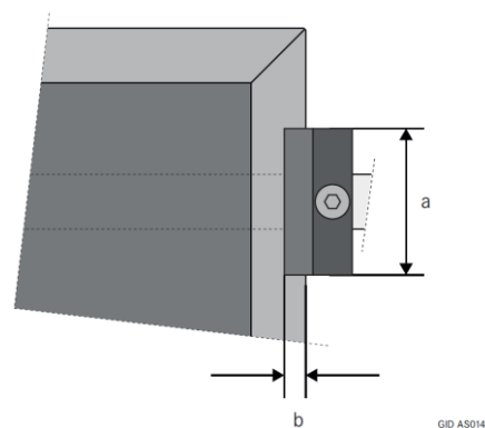
Abb. 8 Definition von Klemmlänge und Klemmtiefe bei gerahmten Modulen
