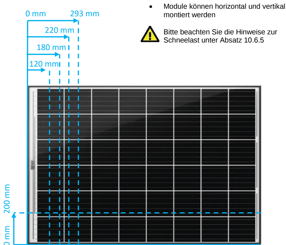
Abb. 10 Montage X61/ X81 Modul mit Klemmen
