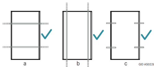
Abb. 3 Zulässige Führung der Montageprofile
