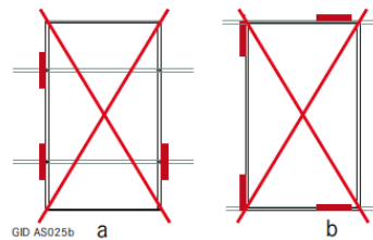
Abb. 6 Unzulässige Anordnung der Klemmen bei gerahmten Modulen (1)
