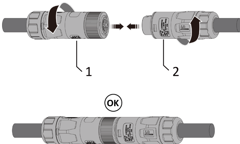
Abb. 28. Bypass Anschluss
