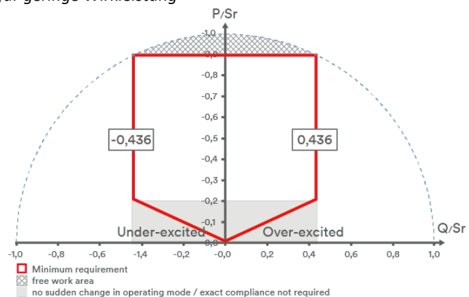
Abb. 198. Auswahl von Min. Cos-phi
