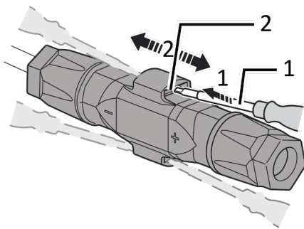
Abb. 246. Steckverbinder abstecken
