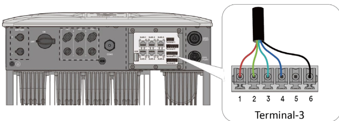
Abb. 60. Netzwerkkabel anschließen
