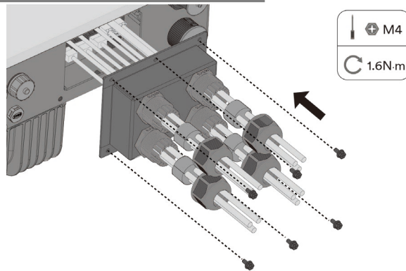
Abb. 54. Befestigen Sie die AC/COM-Abdeckung
