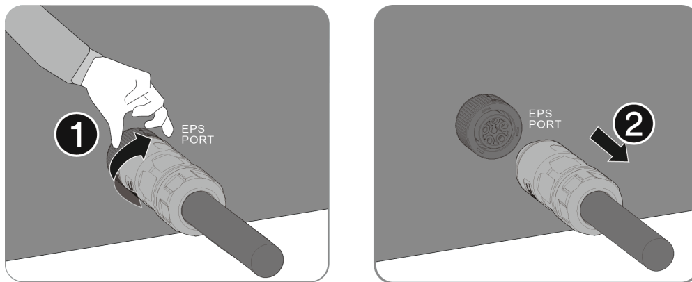
Abb. 243. Lösen und entfernen Sie den Backup-Anschluss.
