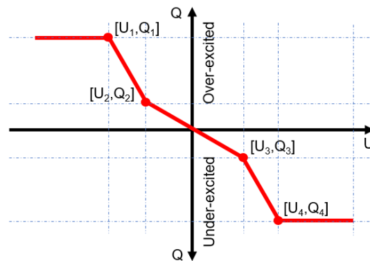
Abb. 194. Wählen Sie „Q(U)-Einstellungen“
