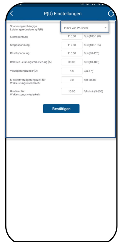
Abb. 180. Wählen Sie die P(u)-Parameter
