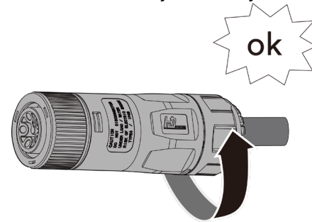
Abb. 17. L1-L3 & N+PE einführen und festziehen
