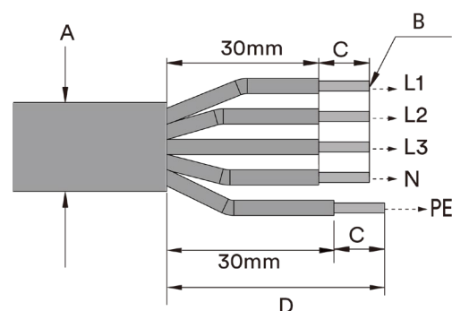
Abb. 15. Isolieren Sie die Drähte ab.
