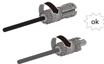
Abb. 40. Kabelverschraubung festziehen
