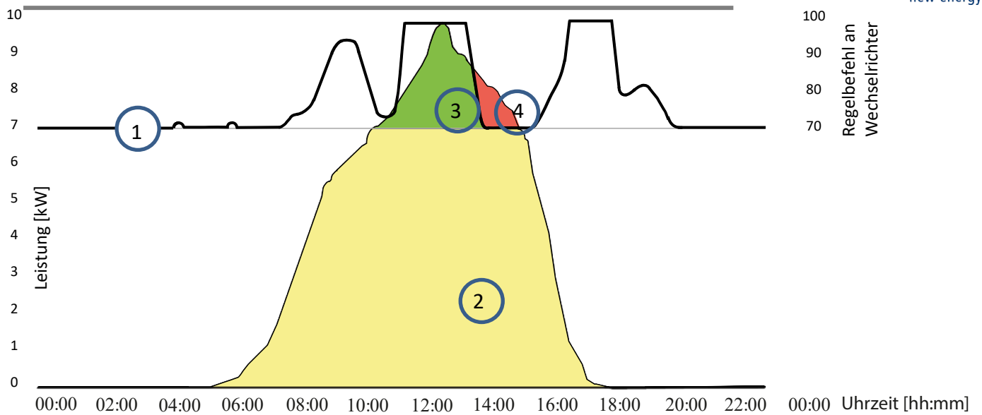
Abb. 238. Diagramm zum Anstieg des Eigenverbrauchs
