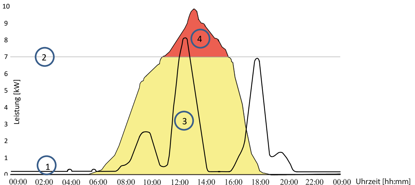
Abb. 237. Diagramm zum Vergleich zwischen Energiebedarf Einfamilienhaus und PV-Leistung
