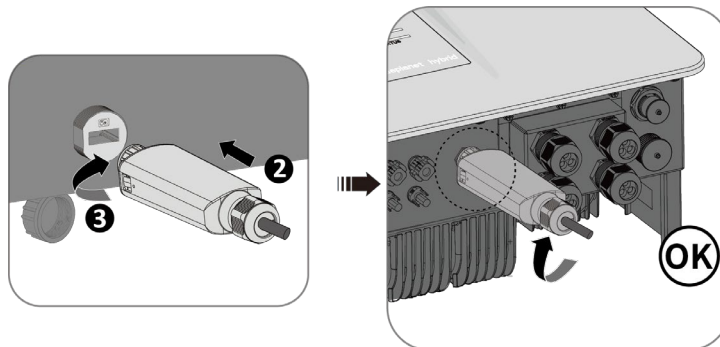
Abb. 48. Verbinden der Kommunikationseinheit (Connect-NH)
