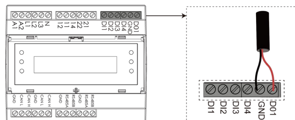
Abb. 59. Verbinden Sie das Netzkabel mit dem Powador-protect
