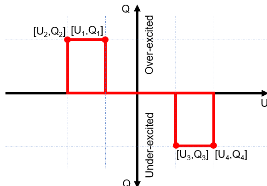
Abb. 197. Q(U)-Kurve und Hysteresis
