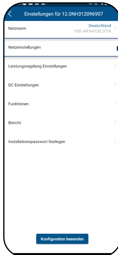
Abb. 146. Wählen Sie Netz-Einstellungen
