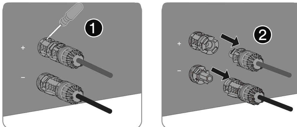
Abb. 244. Lösen und entfernen Sie den PV- /Batterie-Anschluss.
