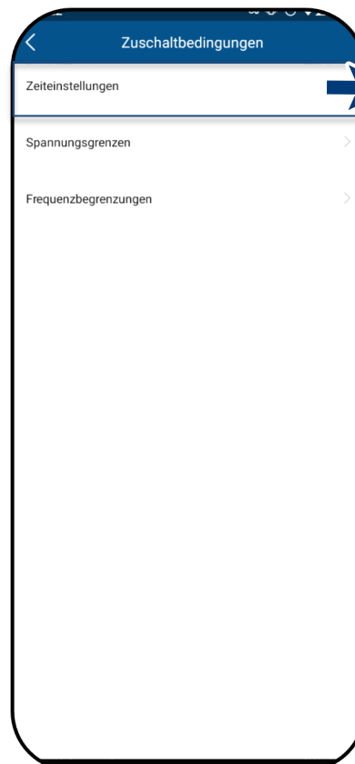
Abb. 144. Wählen Sie die Zeiteinstellungen.
