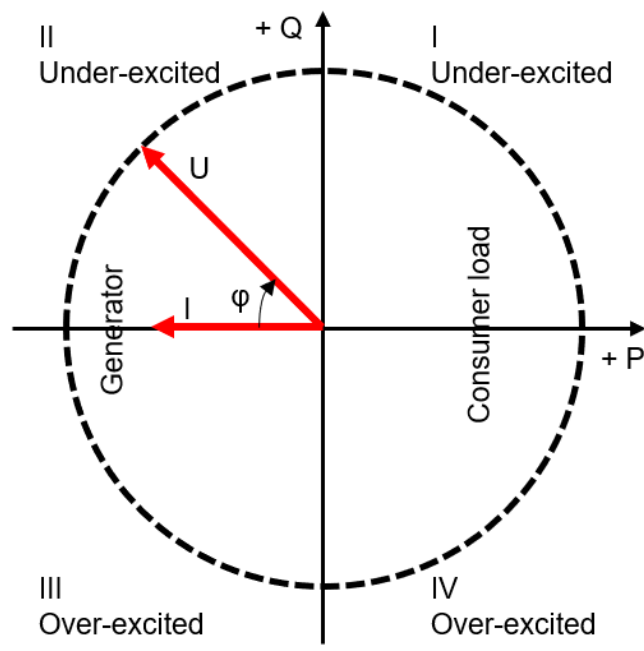
Abb. 186. Lastreferenz-Pfeilsystem
