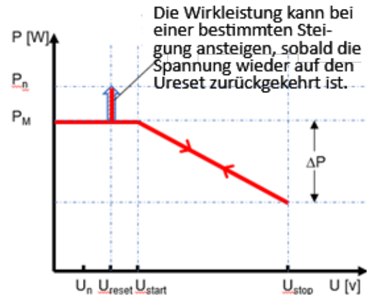
Abb. 181. Nicht-Hysterese
