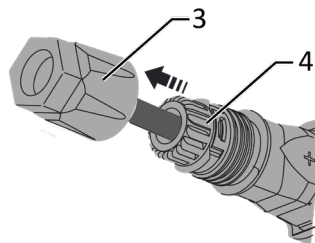
Abb. 30. Einsatz in Hülse schieben
