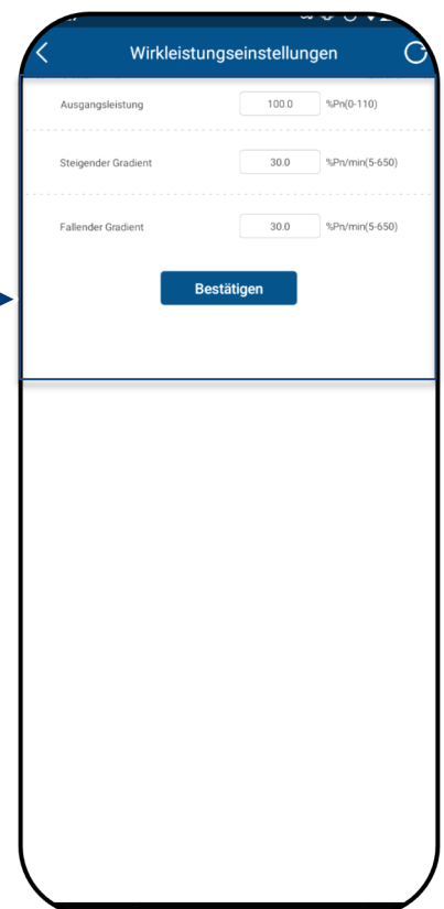
Abb. 203. Definieren der max. Wirkleistung (AP) und Gradienten
