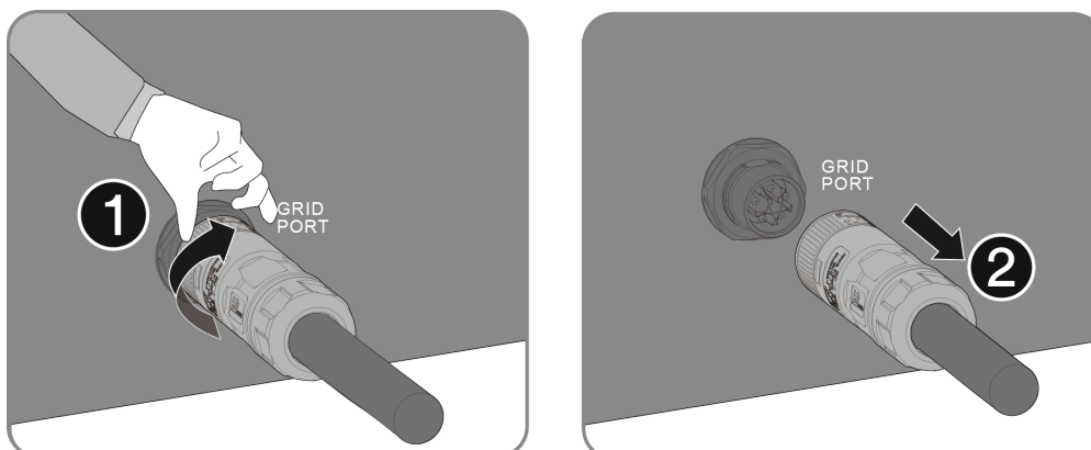
Abb. 242. Lösen und entfernen Sie den AC-Anschluss.
