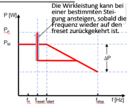
Abb. 177. Hysterese
