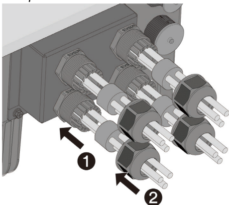
Abb. 55. Mutter anziehen
