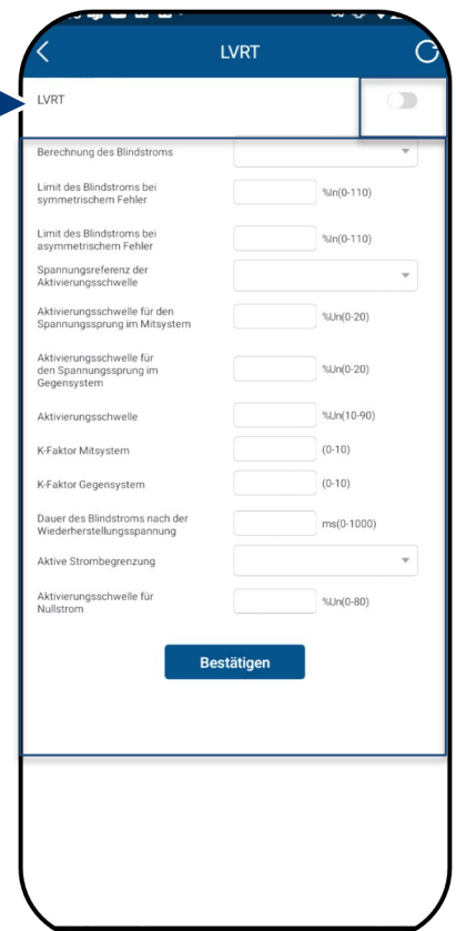
Abb. 168. Einstellen der LVRT-Parameter
