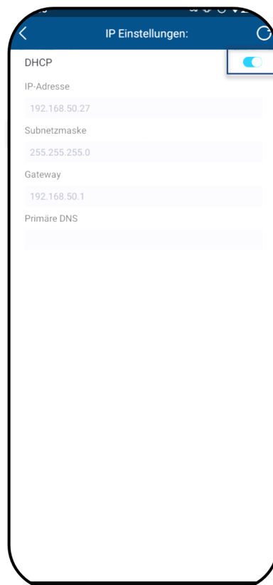
Abb. 87. DHCP deaktivieren
