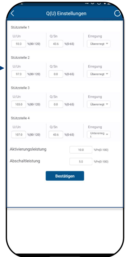
Abb. 195. Bestimmen Sie die Q(U)-Parameter
