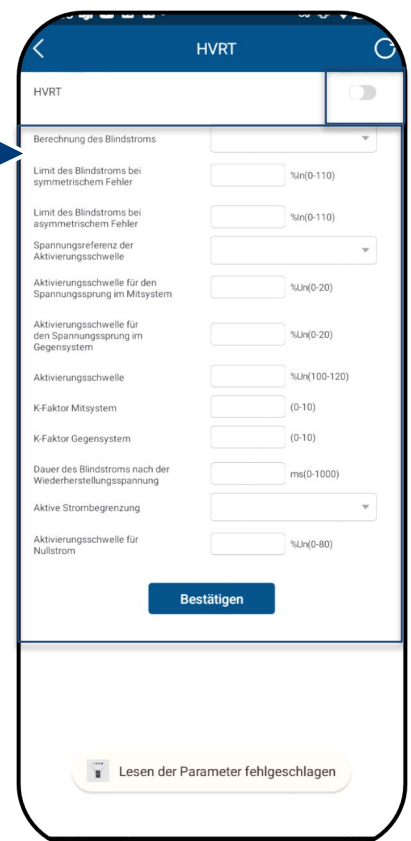
Abb. 172. Einstellen der HVRT-Parameter
