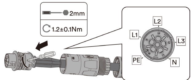
Abb. 24. Kabel am Kontaktträger befestigen
