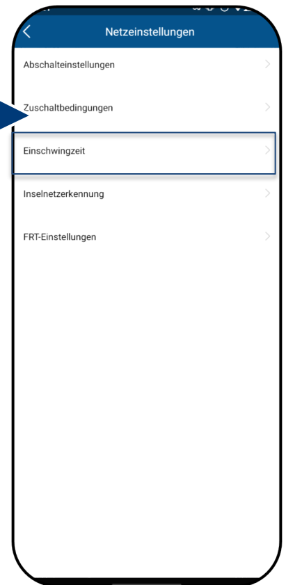
Abb. 155. Wählen Sie Einschwingzeit
