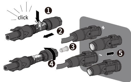
Abb. 35. Setzen Sie die DC-Steckverbinder ein und verschließen Sie ungenutzte Steckverbinder
