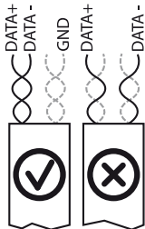
Bild 13: Adernverdrillung
