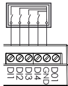
Bild 10: Rundsteuerempfänger
