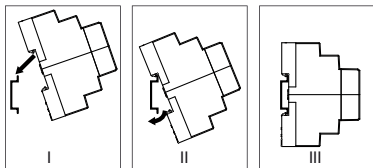
Bild 2: Hutschienenmontage
