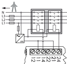
Bild 9: DC-versorgte Kuppelschalter
