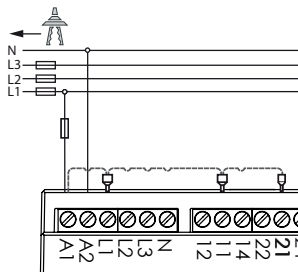
Bild 5: AC-Anschluss mit Drahtbrücke
