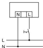
Standardbetrieb mit Ein-/Ausschalter (OF/OFL 120 - 240)
