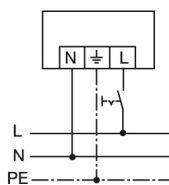
Standardbetrieb mit Ein-/Ausschalter (OF/OFL 500)
