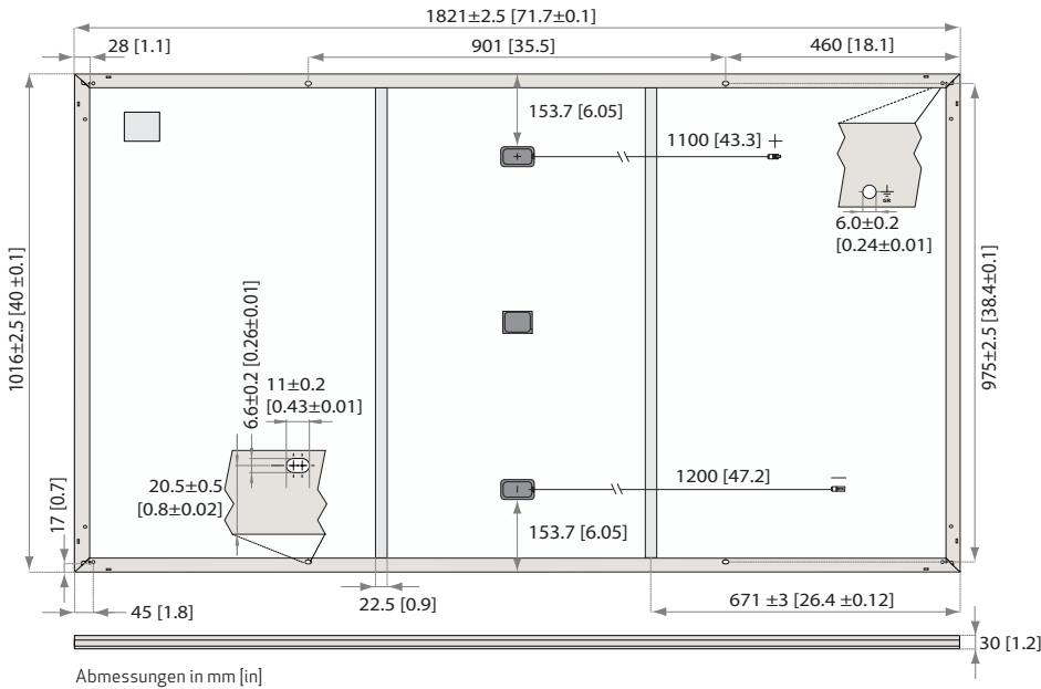
Abb. 21: Abmessungen: REC Alpha Pure Serie
