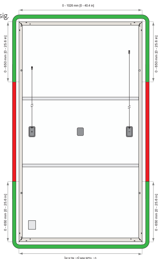
Abb. 24: MLPE-Geräte Installationsbereiche: REC Alpha 72 Serie
