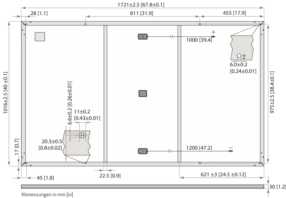
Abb. 19: Abmessungen: REC Alpha Serie
