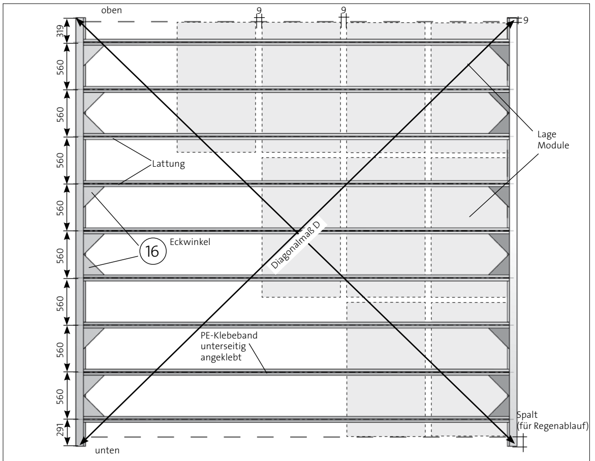
Abb. C 3-7 Ansicht Trägerrost von unten
