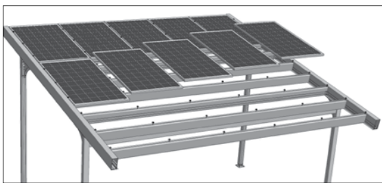
Abb. C 5-3 Montage 2. Reihe
