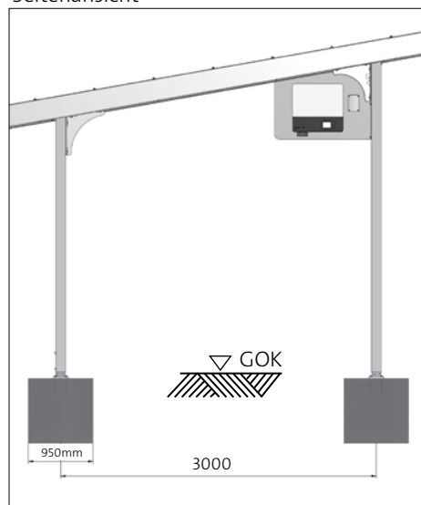
Abb. C 1-1 Maße Fundamente [mm]
