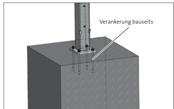
Abb. C 1-4 Fundamentadapter auf Fundament
