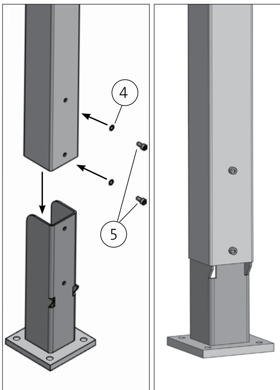
Abb. C 2-2 Fundamentadapter/ Stützprofil
