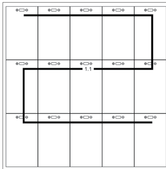
Abb. C6-1 Verschaltungsplan Module
