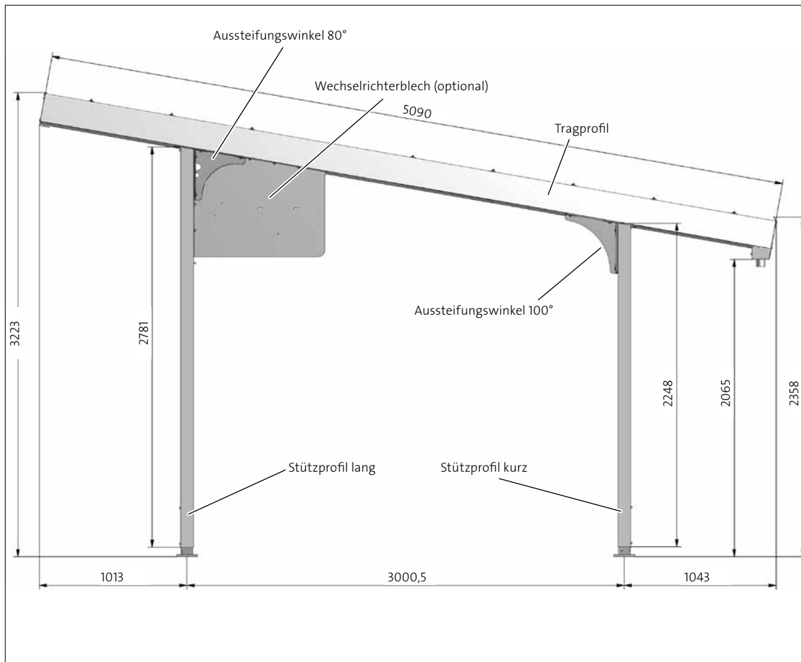
Abb. C 2-14 Übersicht Seitenteil nach der Montage
