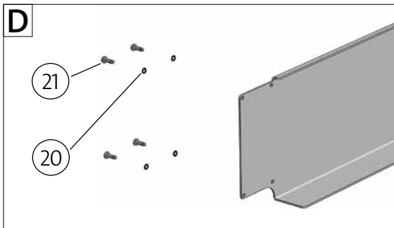
Abb. B 2-5 Anschluss Stirnblech
