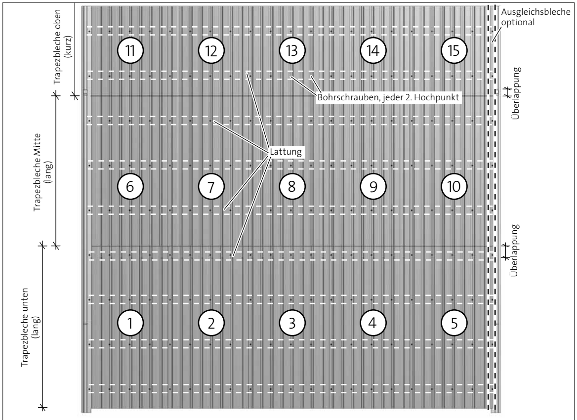
Abb. C 7-4 Ansicht Trapezbleche von unten
