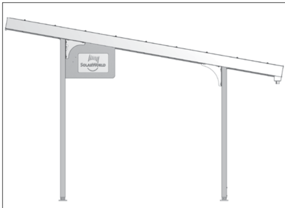
Abb. C 2-1 Seitenansicht montiertes Seitenteil
