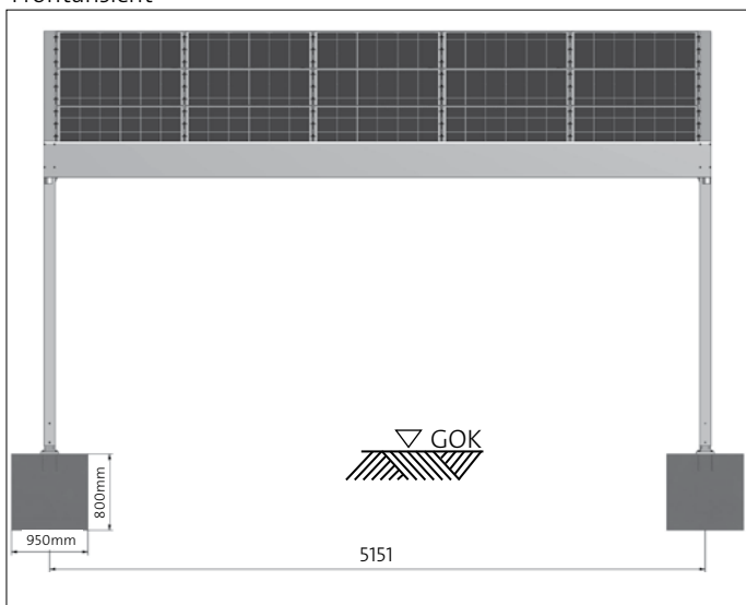
Abb. C 1-2 Maße Fundamente [mm]
