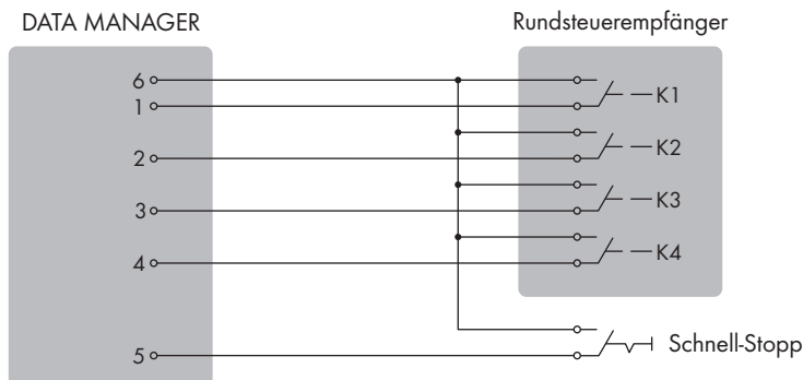
Abbildung 7: Anschluss eines Rundsteuerempfängers
