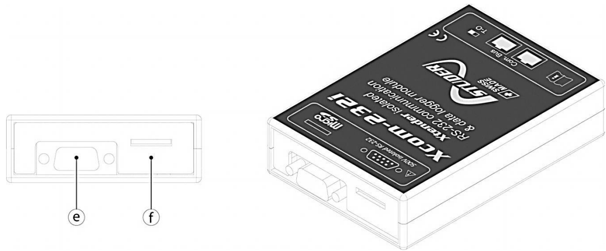
Abbildung 4.2: Rück- und isometrische Ansicht des Xcom-232i
