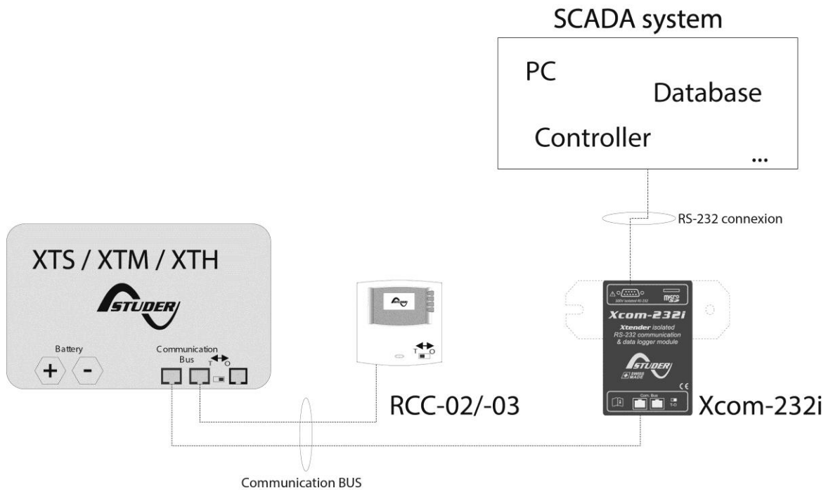
Abbildung 3.1: Anschlussschema des Xcom-232i (Beispiel 1)
