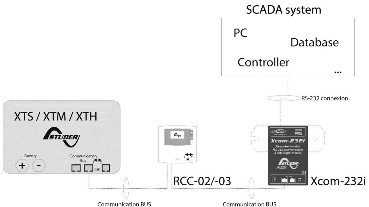
Abbildung 3.2: Anschlussschema des Xcom-232i (Beispiel 2)
