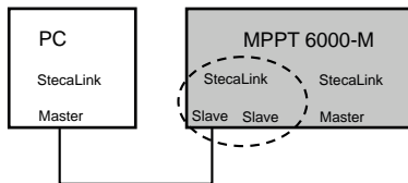
Abb. 10: Beispiel Anschluss PC an MPPT 6000-M, z. B. für Update-Funktion
