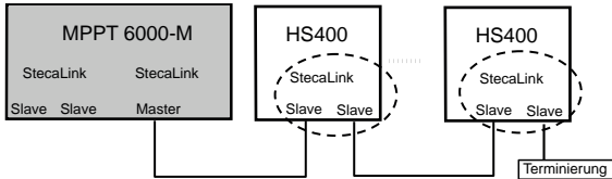
Abb. 9: Beispiel Busverkabelung mit MPPT 6000-M und zusätzlichen PA HS400-Stromsensoren
