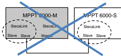
Abb. 11: Verbindung MPPT 6000-M Slave-Anschluss mit weiteren Slave-Anschlüssen von MPPT 6000-S oder PA HS400 nicht erlaubt
