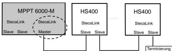
Abb. 13: Beispiel Busverkabelung mit MPPT 6000-M und zusätzlichen PA HS400-Stromsensoren
