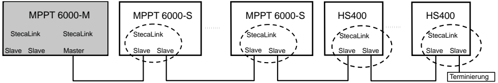
Abb. 8: Beispiel Busverkabelung mit MPPT 6000-M, MPPT 6000-S und PA HS400-Stromsensoren
