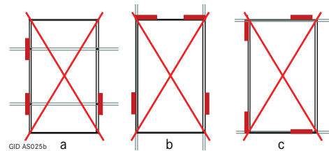
Abb. 6 Unzulässige Anordnung der Klemmen bei gerahmten Modulen (1)
