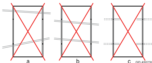
Abb. 4 Unzulässige Führung der Montageprofile
