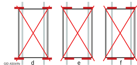
Abb. 7 Unzulässige Anordnung der Klemmen bei gerahmten Modulen (2)
