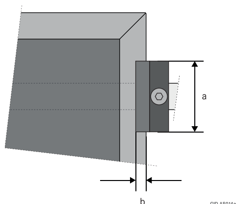
Abb. 8 Definition von Klemmlänge und Klemmtiefe bei gerahmten Modulen
