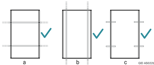
Abb. 3 Zulässige Führung der Montageprofile
