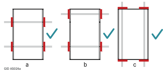
Abb. 5 Zulässige Anordnung der Klemmen bei gerahmten Modulen
