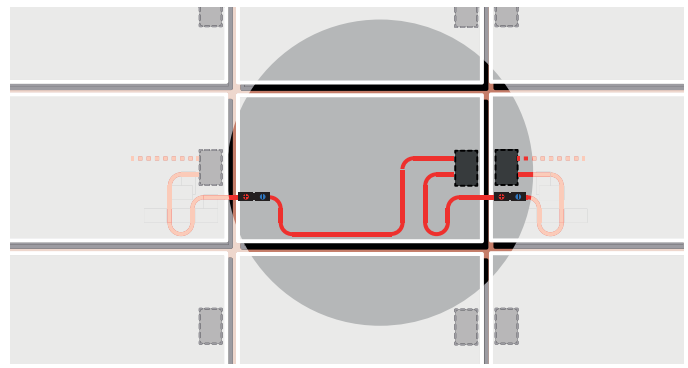
Abb. 2 U-förmige Leitungsführung an Anschlussdose bei Quermontage
